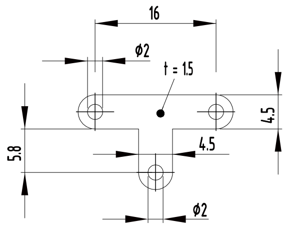
Detailansicht Steuerhebel (2:1)
