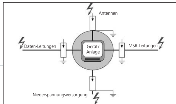
Bild 6: Geräte bzw. Anlagen haben Verbindungen zu verschiedenen Systemen – welche jedes für sich zu schützen ist
