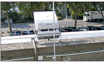
Bild 4: Fehlerhafte Anordnung einer Fangstange
