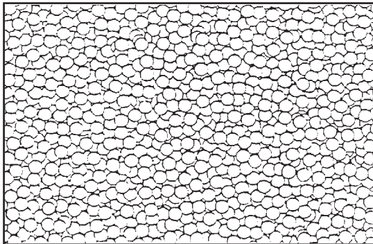
Abb. 3: Mesmers Modell einer aus gleichförmigen, in ungeordneter dichtester Packung befindlichen „Urkügelchen“ aufgebauten Ätherflüssigkeit. Diese Ursubstanz alles Seienden haben wir uns im Grundzustand in permanenter ungeordneter Strömungsbewegung vorzustellen.
