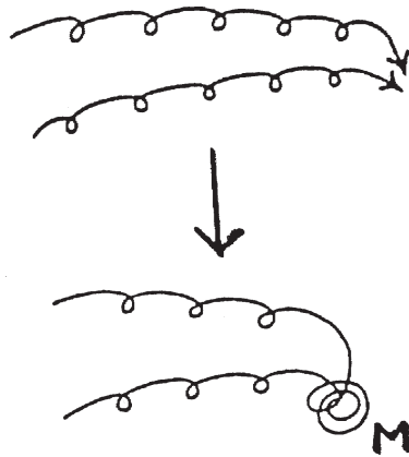
Abb. 1: Die nach Reich einer kosmischen Liebesfunktion entsprechende Vereinigung zweier Orgon-Energie-Ströme zu einer Wirbelstruktur. M = Primordiales Masseteilchen.
