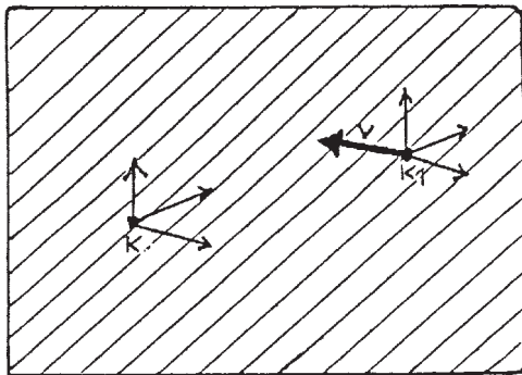
Abb. 19: Ein ruhendes ( K ) und ein bewegtes ( K_1 ) Bezugssystem im klassischen Äthermodell.
