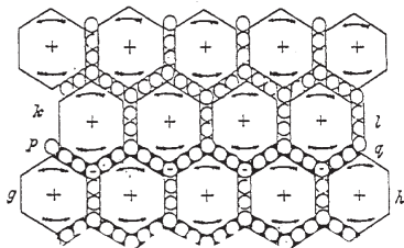
Abb. 8: Maxwells Äthermodell des Magnetismus. Die mit + bezeichneten sechseckigen Zellen im oberen Bildteil stellen einen schematischen Querschnitt durch gleichsinnig rotierende
