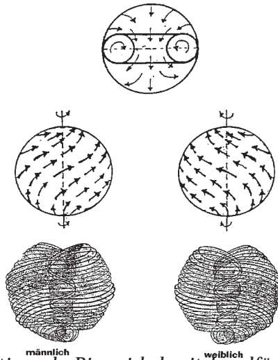
Abb. 15: Der rotierende Ringwirbel mit kugelförmig ergänzter Strömungshülle. Die Strukturvariante links stellt im Kosmonenmodell ein Elektron dar, diejenige rechts ein Positron. Darunter Babbitts Originaldarstellung der weiblich-männlichen Urpolarität der Materie.
