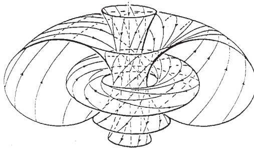
Abb. 21: Darstellung eines Elementarteilchens nach der Twistor-Theorie des Relativitätstheoretikers Penrose. Die dargestellten Strömungslinien stellen hier allerdings nicht einen Ätherwirbel, sondern eine rein mathematisch-geometrische Feldkonfiguration dar.
