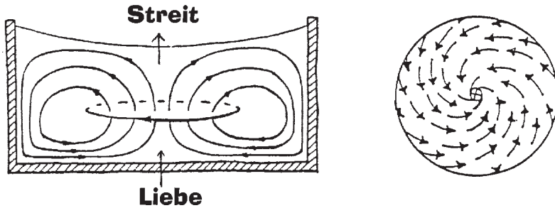
Abb. 17: Empedokles Vorstellung der beiden polaren, seelisch-lebendigen Grundkräfte der Natur (Liebe und Streit) als ein- und ausströmender Pol eines rotierenden Ringwirbels in einer Flüssigkeit. Rechts davon Aufsicht auf die dem Liebespol entsprechende, als zentripetaler, antigravitationeller Sog wirkende Spiralströmung an der Unterseite des rotierenden Ringwirbels.
