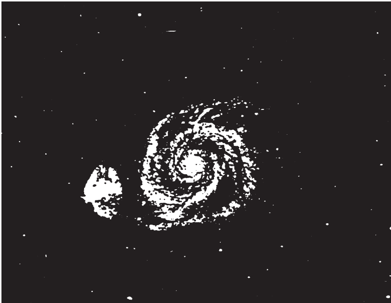
Abb. 2: Die Spiralgalaxis Messier 51
