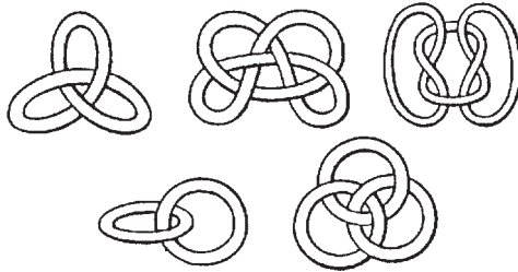
Abb. 13: Beispiele für Lord Kelvins aus untereinander verflochtenen Ringwirbeln im Äther bestehende Atommodelle. Die aus zwei Ringwirbeln aufgebaute Struktur links unten sollte z. B. dem Natrium-Atom entsprechen.
