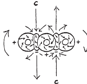
c = das Proton mit Lichtgeschwindigkeit durchfließender Aetherstrom.
