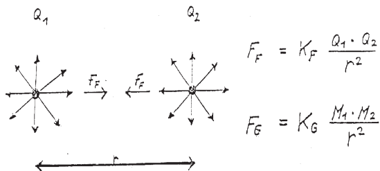
Abb. 5: Anziehende Wechselwirkung F_F zweier punktförmiger Quellen mit der Ergiebigkeit Q_1 bzw. Q_2 , die sich im Abstand r in einem flüssigen Medium befinden: F_F = K_F \cdot Q_1 \cdot Q_2 / r^2 ( K_F = vom Fluidum abhängige Konstante) F_G : Völlig analoge Formel für die Gravitationskraft zwischen zwei Massen M_1 und M_2 .
