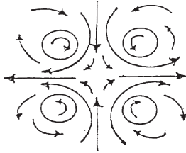
Abb. 10: Zweidimensionale Darstellung einer aus vier Wirbelelementen aufgebauten symmetrischen Strömungsstruktur. Diese im Äthermodell einem neutralen Massepartikel entsprechende Struktur wird durch die parallele Strömungsrichtung ihrer unmittelbar benachbarten Wirbelelemente stabilisiert und weist je zwei einander gegenüber liegende ein- und ausströmende Pole auf.
