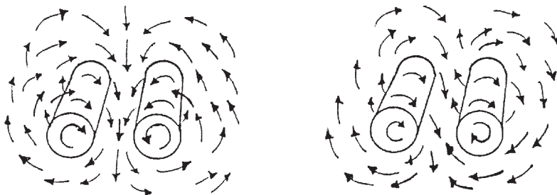
Abb. 7: Anziehende oder abstoßende Wechselwirkung zweier in einer Flüssigkeit nebeneinander gegensinnig oder gleichsinnig rotierender Zylinder nach Weyher und Bjerknes.
