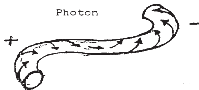
Abb. 24: Darstellung des sich durch den Raum bewegenden Photons im Kosmonenmodell als wellenförmige, aus je einem halben Elektron- und Positron-Ring bestehende Strömungsstruktur.
