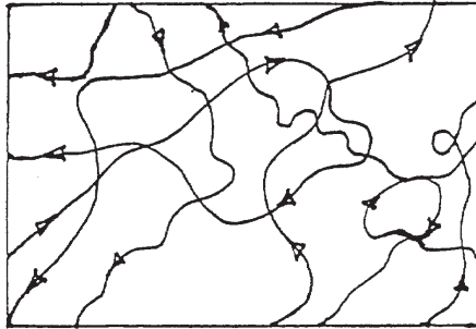
Abb. 20: Schematische Darstellung möglicher Bahnkurven einzelner Kosmonen im unstrukturierten Grundbewegungszustand des Zeit-Raumes, von einem beliebigen Bezugskörper aus betrachtet.
