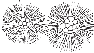
Abb. 4: Von ein- und ausströmenden Ätherstrahlen durchströmte Atome in Mesmers Originaldarstellung. Die den subatomaren Kernbausteinen entsprechenden Kugelemente hat man sich als kugelförmige Agglomerationen von Ätherpartikeln vorzustellen.
